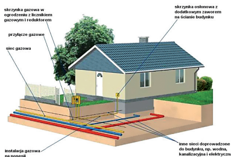
Poglądowy schemat podłączenia gazu
